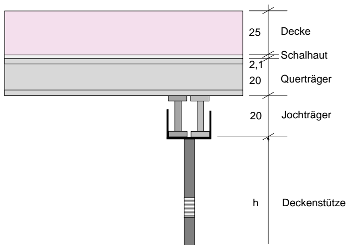
Bild 6.22 Querschnitt Deckenschalung
